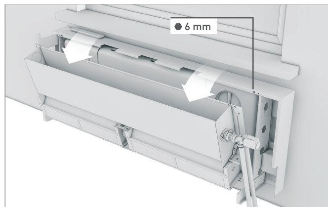
Obróć wentylokonwektor do siebie
