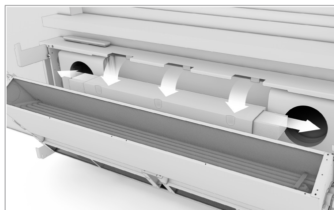
Wymij filtry powietrza odpinając trzy spinki i opuszczając obudowę filtra powietrza do przodu o 90 stopni. Wsuń obydwie filtry z obudowy.
