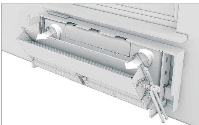
Zdemuj pokrywę, obracając je o ćwierć obrotu w lewo, a następnie pociągając do siebie. Sprawdź czystość i jeśli to konieczne, wyczyść wstępny filtr siatkowy.
